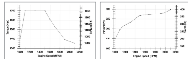
Curvas de Torque y Potencia
